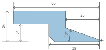
SCHARFSCHIENE 66/24 20° GEKRÖPFT
