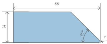
SCHARFSCHIENE 66/24 45°
