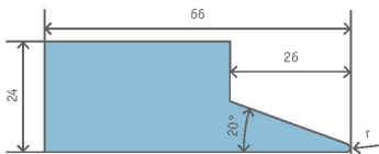
RAIL À ARÊTE VIVE 66/24 20°
