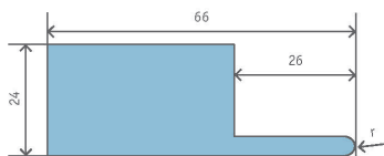
RAIL À ARÊTE ARRONDIE 66/24 R = 1 - 12
