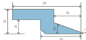
RAIL À ARÊTE VIVE 66/24 20° COUDÉ
