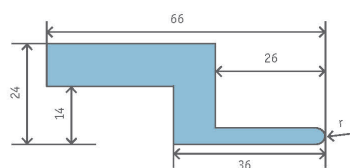
RAIL À ARÊTE ARRONDIE 66/24 LARGE COUDÉ
