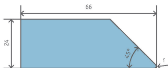
RAIL À ARÊTE VIVE 66/24 45°
