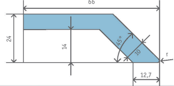
RAIL À ARÊTE ARRONDIE 66/24 LARGE COUDÉ
